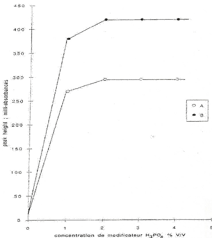
Fig.2[5]. Influența concentrației modificatorului asupra semnalului
